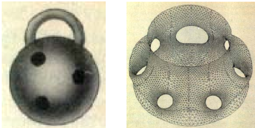
Сфера со три дупки и една рачка и една нејзина тополошка трансформација
