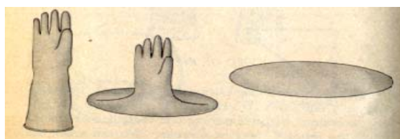
Трансформација на ракавица во диск
