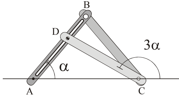
Цртеж 1. Инструмент за трисекција на тапи агли.
